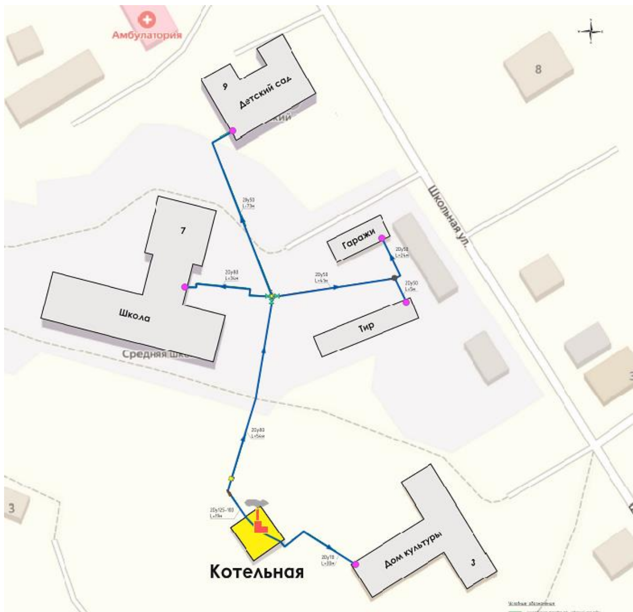
1.3.2.1 Схема тепловой сети от источника тепловой энергии Котельной п. Ручей
